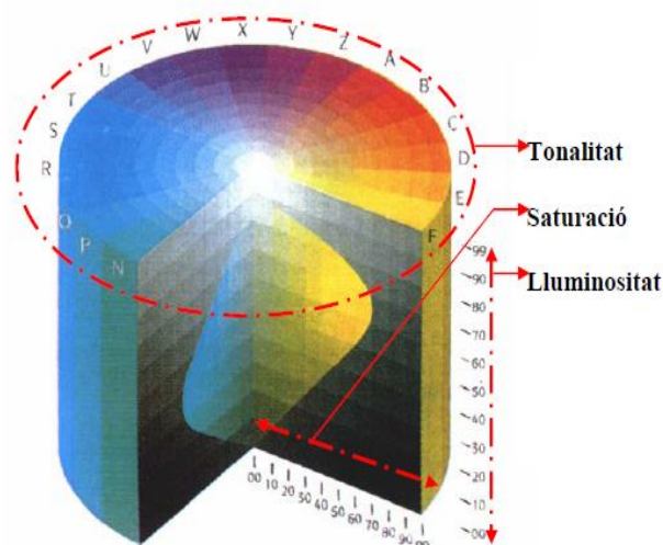
Sistema ACC
