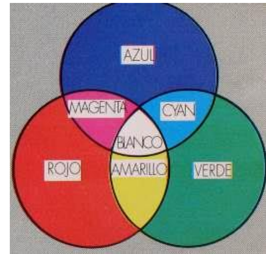
Codificació RGB
