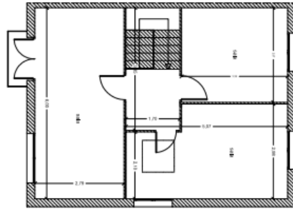
PLANTA PRIMERA
