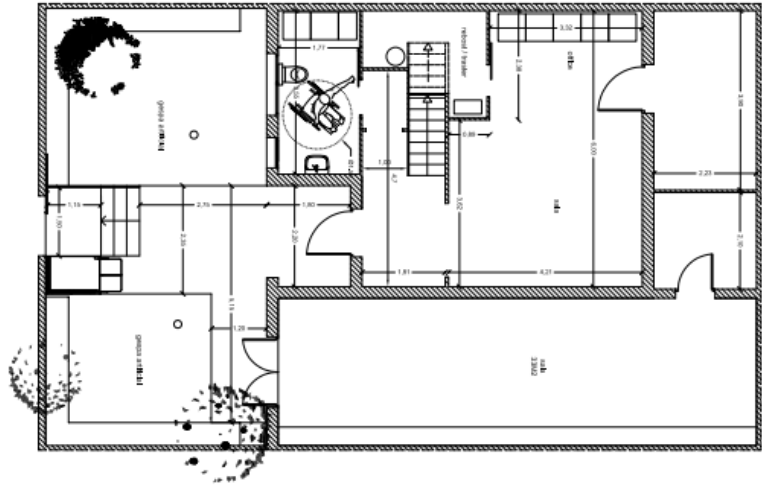
PLANTA BAIXA
