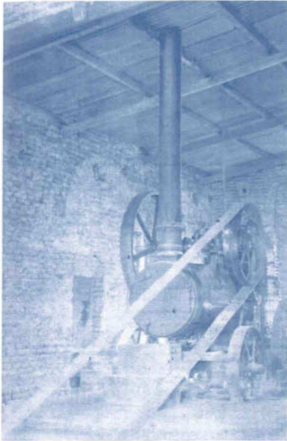
Màquina de vapor alemanya, de 70 HP, de l'estil de "la Chapelle". Cap a l'any 1890
